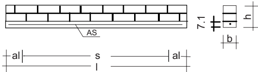
Flachsturzhöhe: 7.1 cm
